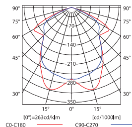
curve of intensity distribution / Lichtverteilungskurve / courbe de répartition de la lumière \eta = 70\%
